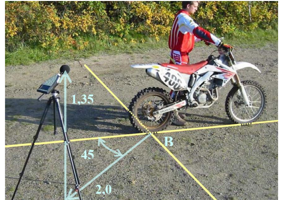
Ljudmätning och kontroll av fordon.
